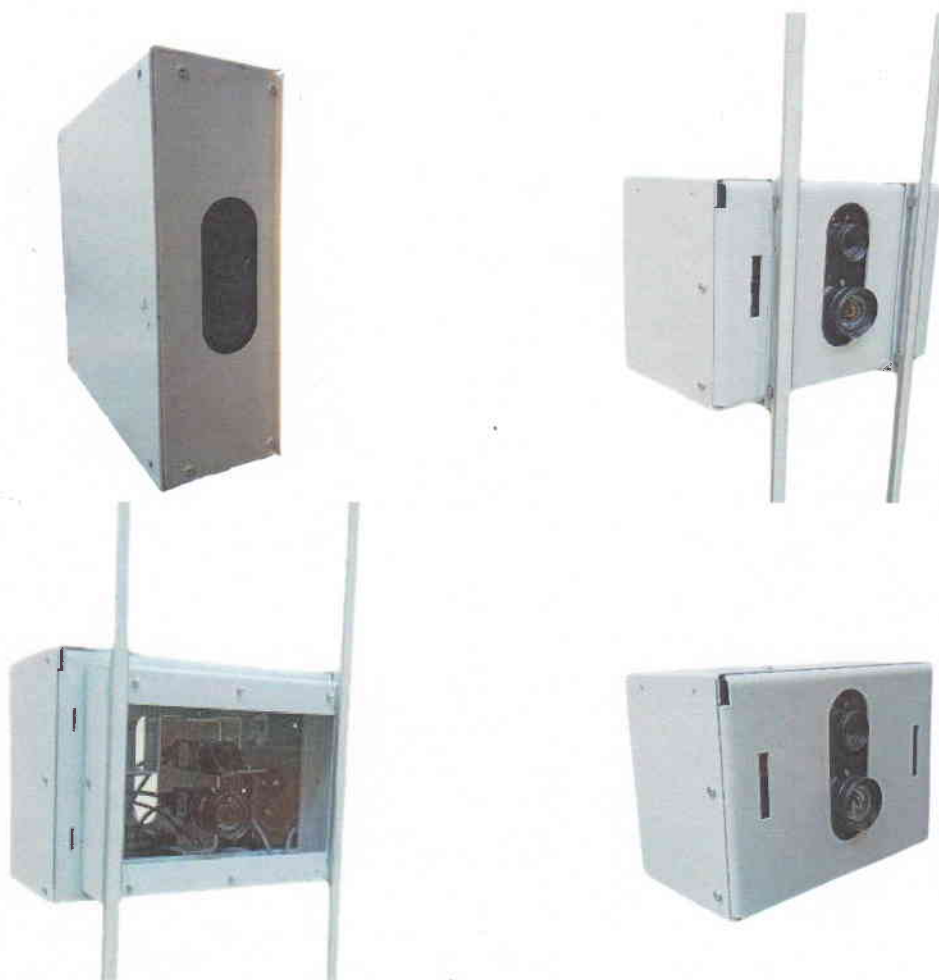
Рисунок 1 - Общий вид систем видеоизмерительных ViEx
